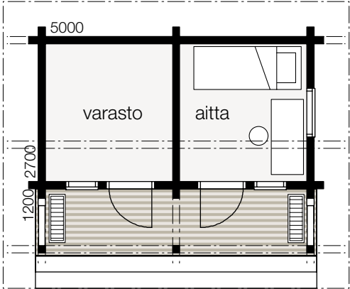
Nalle aitta, kerrosala 14 m² 1:100
