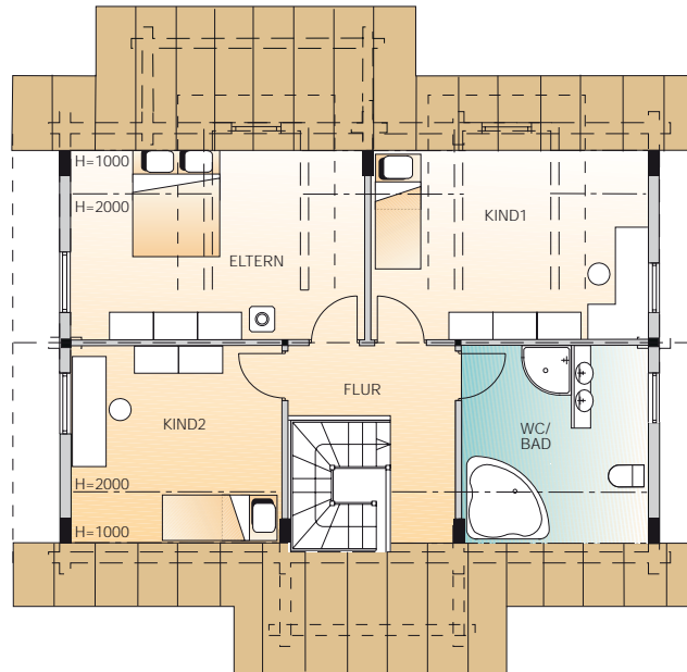
Dachgeschoss 60 m 2 1:150
