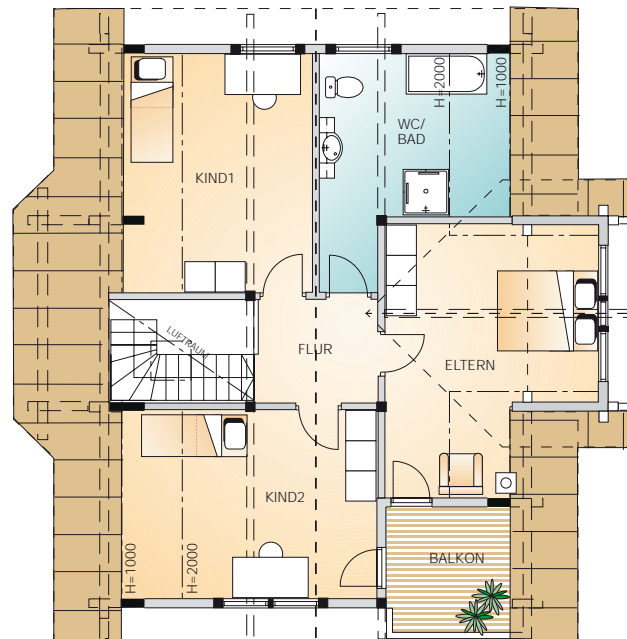
Dachgeschoss 69 m 2 1:150
