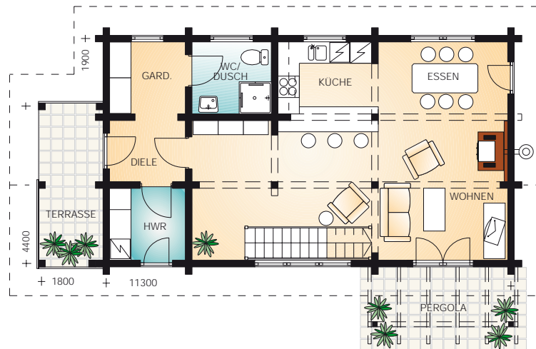
Erdgeschoss 61 m 2 1:150
