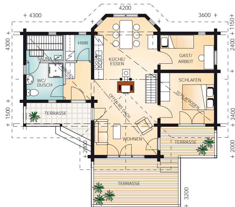
Grundriss 1:150
