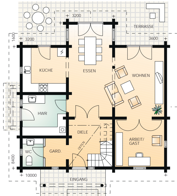
Erdgeschoss 78 m 2 1:150
