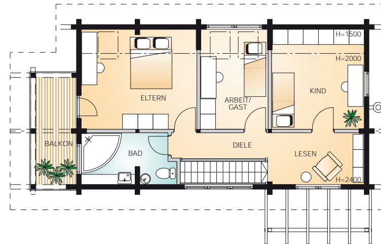
Dachgeschoss 60 m 2 1:150
