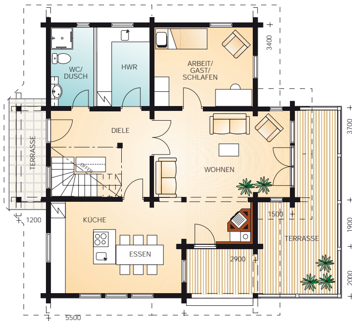
Erdgeschoss 81 m 2 1:150
