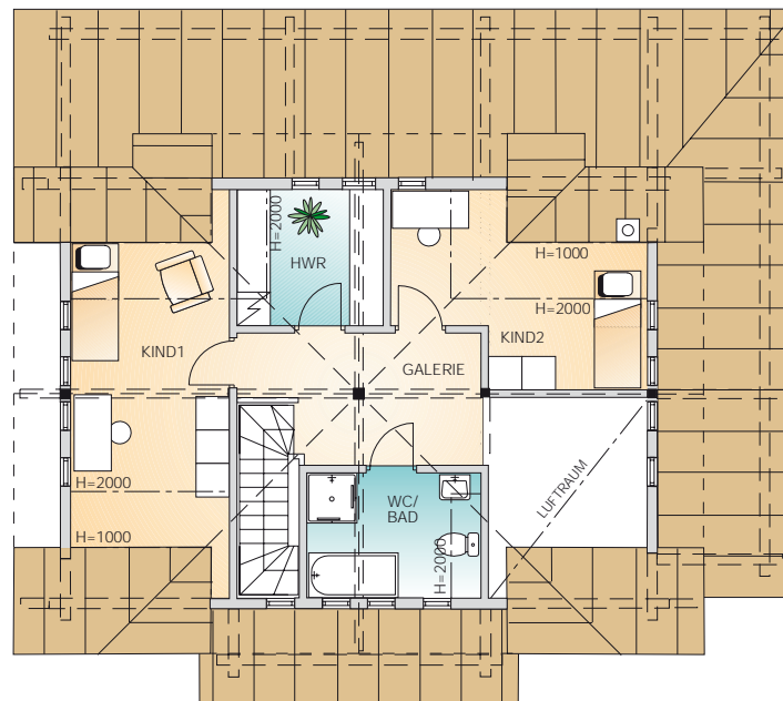
Dachgeschoss 44 m 2 1:150
