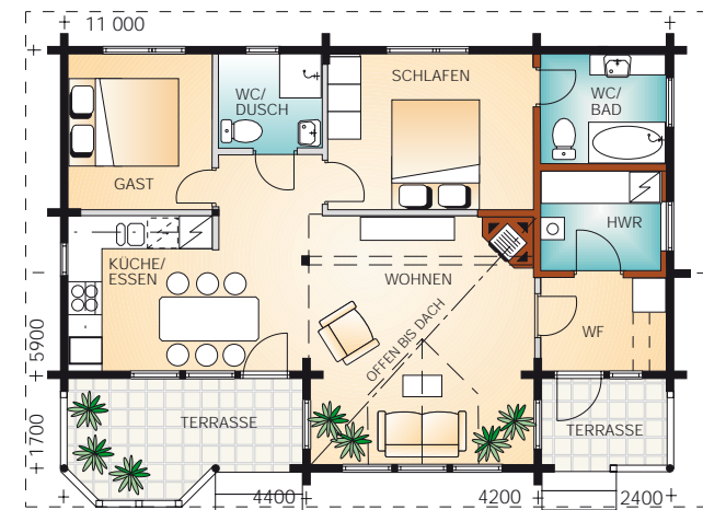
Grundriss 1:150
