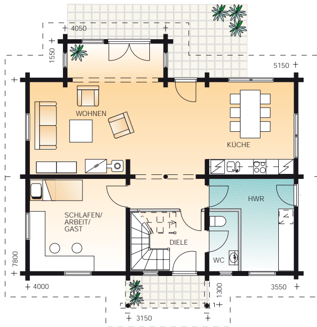
Erdgeschoss 79 m 2 1:150
