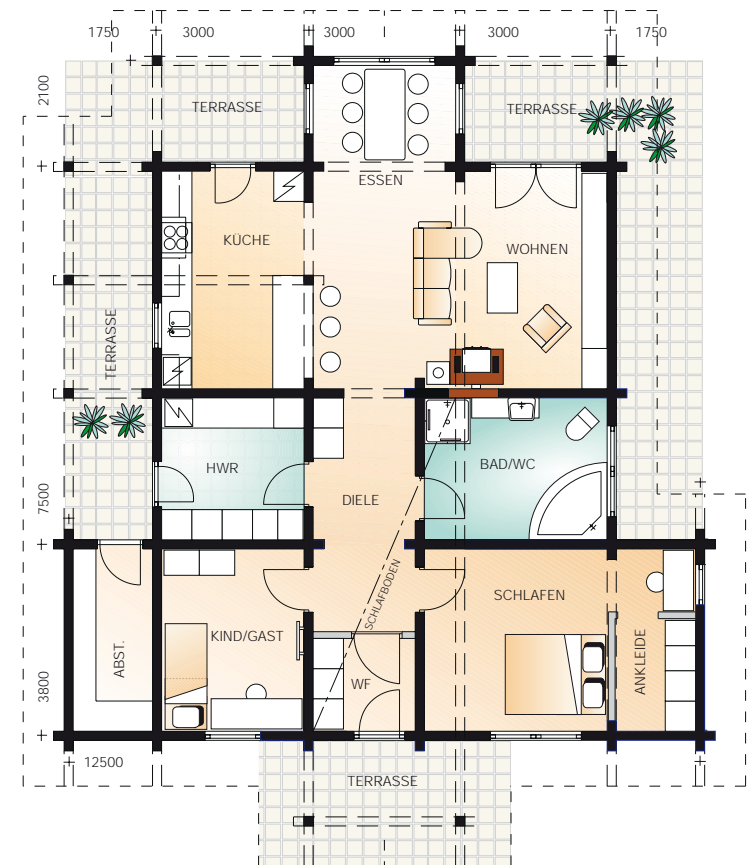
Grundriss 1:150
