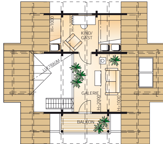
Dachgeschoss 17 m 2 1:150
