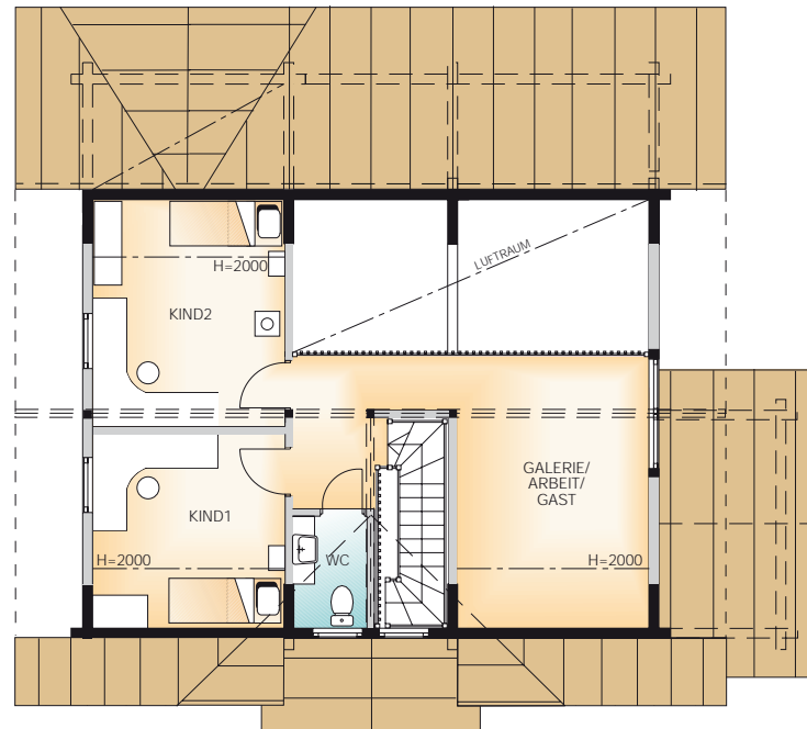
Dachgeschoss 47 m 2 1:150
