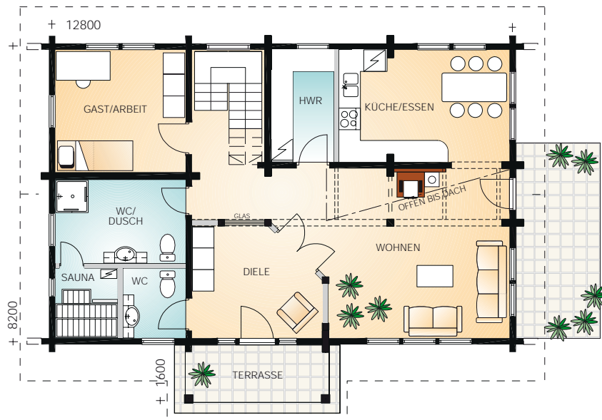
Erdgeschoss 91 m 2 1:150
