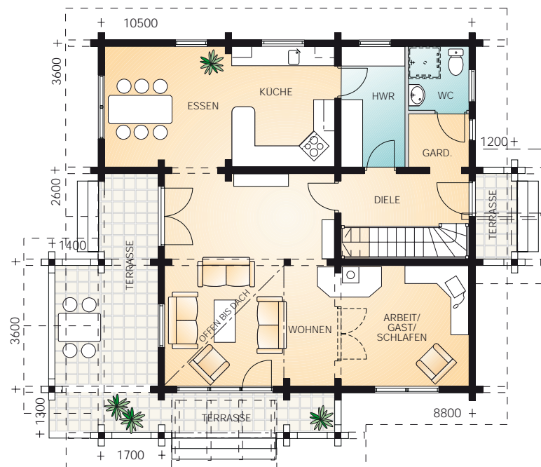
Erdgeschoss 81 m 2 1:150
