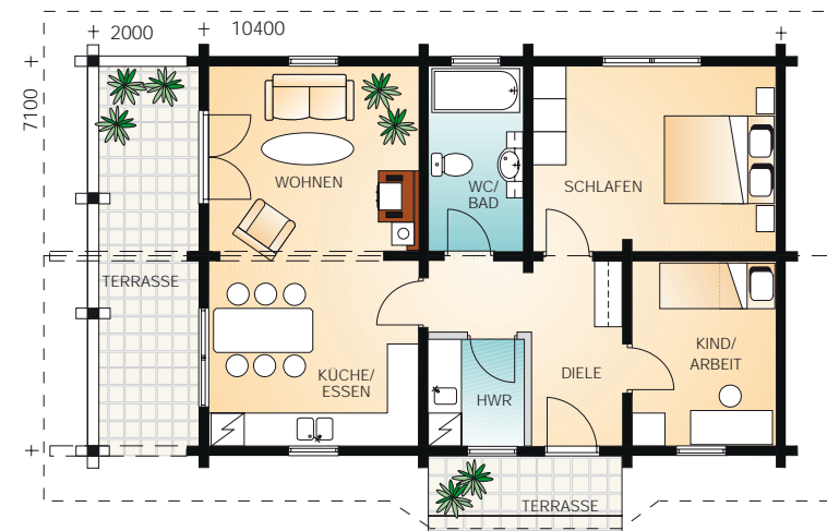
Grundriss 1:150
