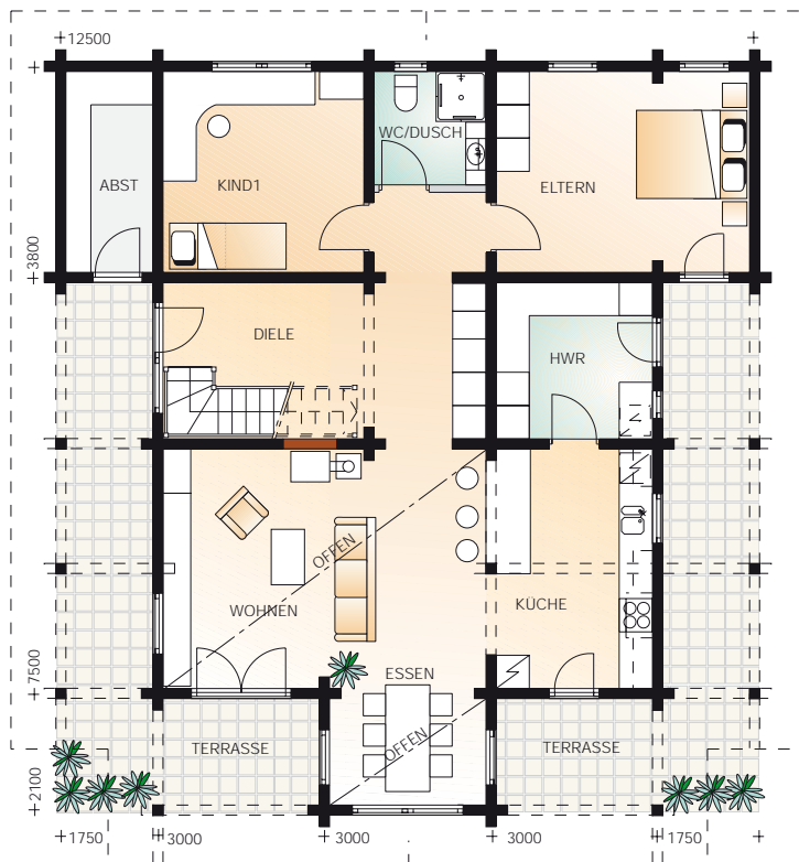
Erdgeschoss 107 m 2 1:150
