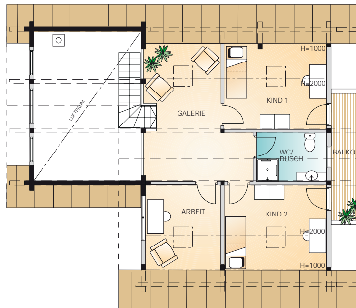
Dachgeschoss 57 m 2 1:150
