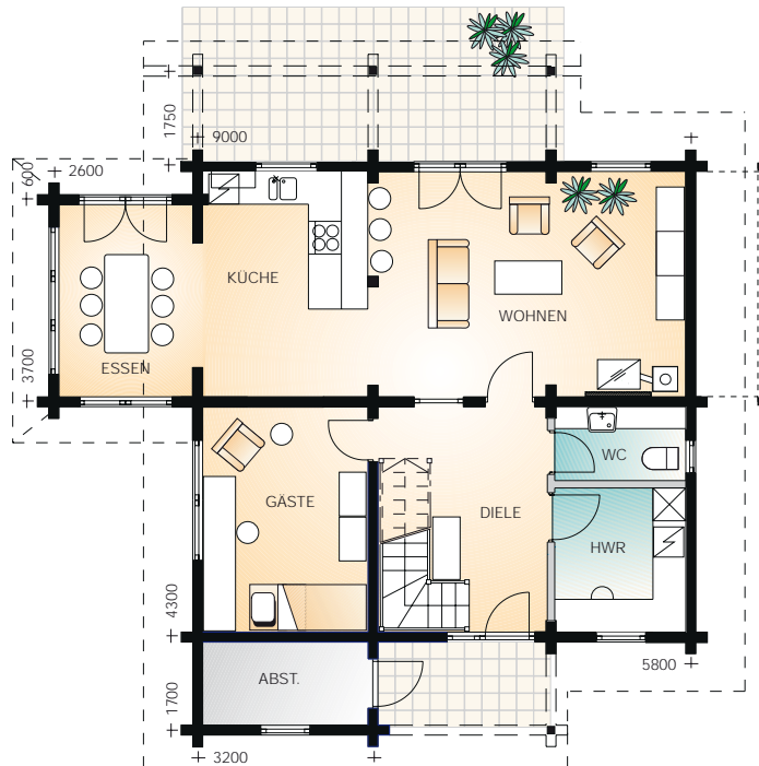
Erdgeschoss 76 m 2 1:150
