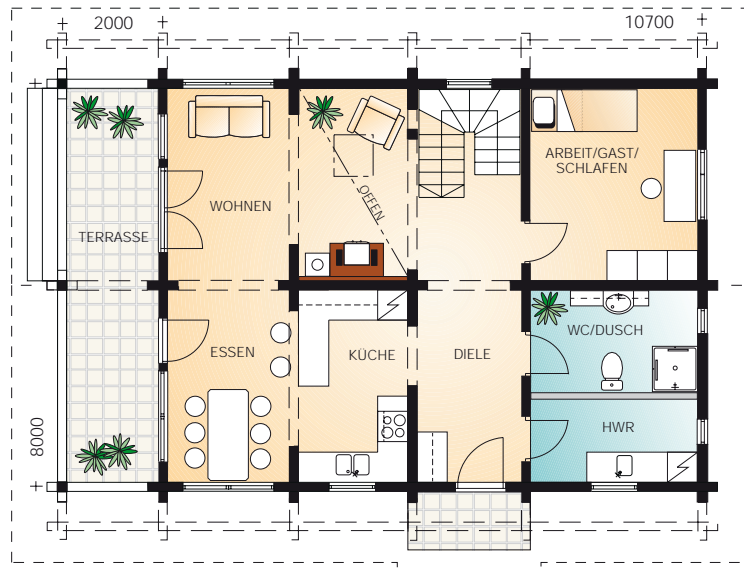
Erdgeschoss 74 m 2 1:150
