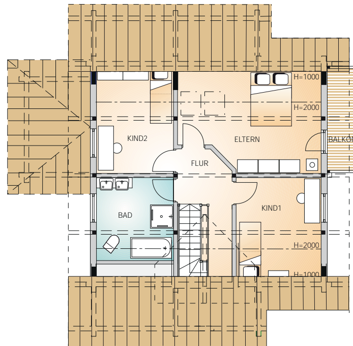
Dachgeschoss 55 m 2 1:150
