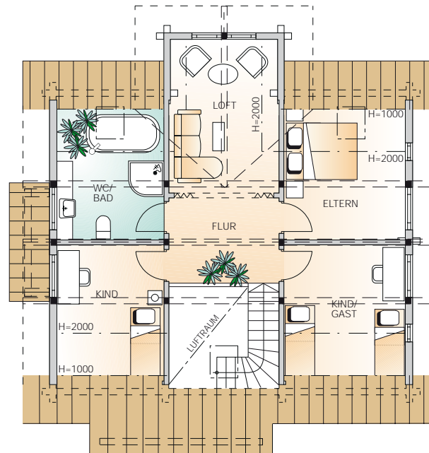
Dachgeschoss 59 m 2 1:150
